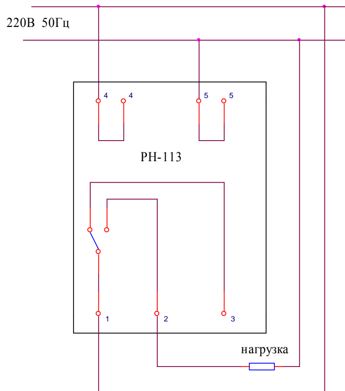
Примечание. Контакты реле показаны при обесточенном реле. Рисунок 2 – Схема подключения реле
