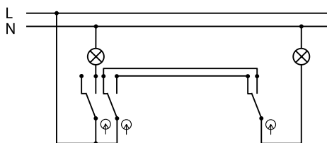
Схема подключения (6+1) 6+6
