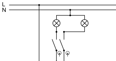
Схема подключения 5
