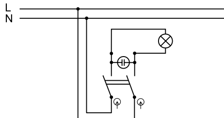
Схема подключения 2S
