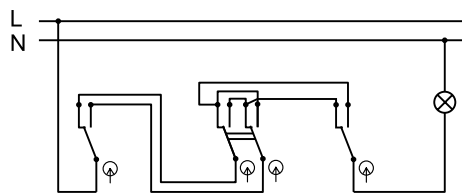
Схема подключения 6 7 6
