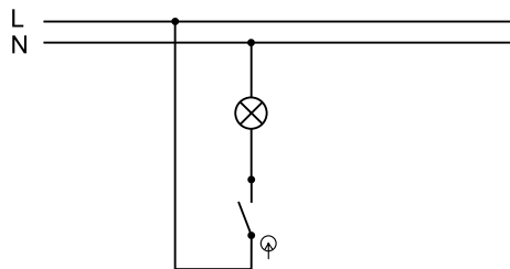
Схема подключения 1
