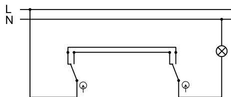
Схема подключения 6 6
