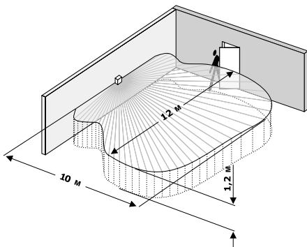
Датчик движения
